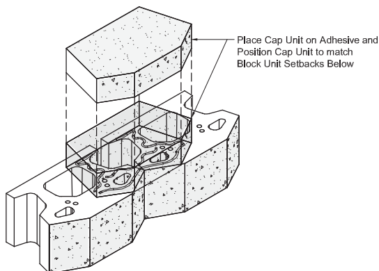
FIGURE I:1 - SECURE THE CAPS
